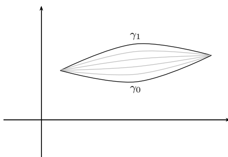
SLIKA 1.8. Homotopija med potema \gamma_0 in \gamma_1
