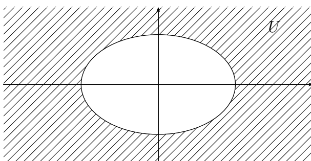
SLIKA 1.10. Odprta okolica U točke \infty
